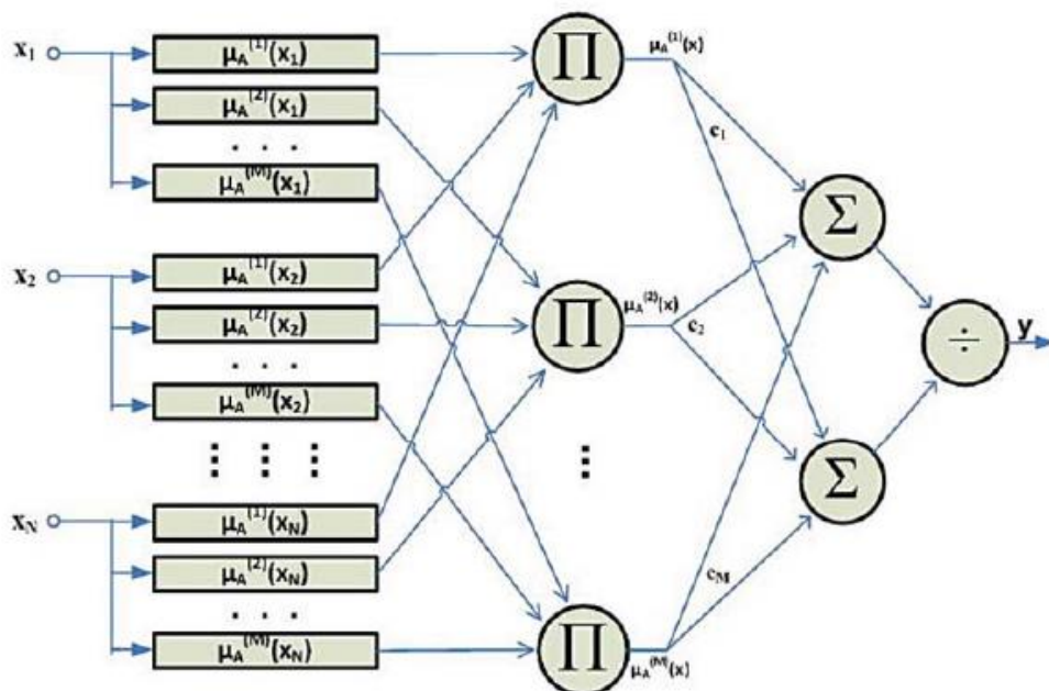
Рисунок 1.5 – Нейро-нечёткая сеть Ванга-Менделя [6]
