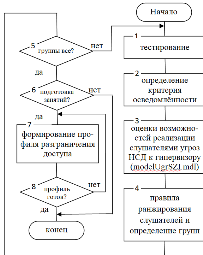
Рисунок 3.16 – Алгоритм функционирования средства оценки динамики состояния информационной системы обучения с информацией специального назначения в условиях угроз НСД с целью автоматизации процесса создания профилей по разграничению профилей на основе технологии «тонкий клиент»
