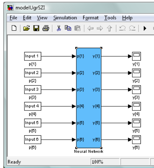
Рисунок 3.1 – Общий вид нейронечёткой модели оценивания возможностей реализации 2 угроз НСД к гипервизору через виртуальные машины в ОИСИЧ (modelUgrSZI.mdl)
