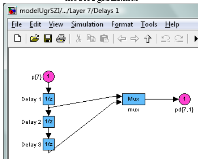
Рисунок 3.11 – Описание задержки выполнения заключительного этапа
