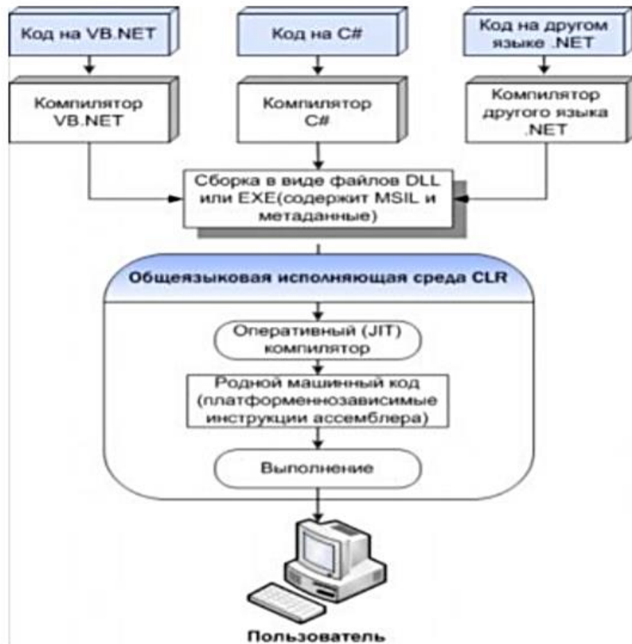
Рисунок 2.1 – Схема общезыковой исполняющей среды и её связи с деассемблированием [83]
