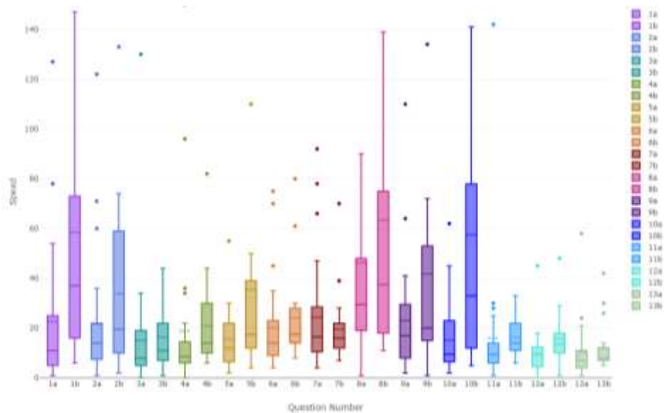
Рисунок 35 – Тест 1: скорость выполнения заданий в секундах для исправленного интерфейса, где a – сенсорные экраны, b – традиционный интерфейс
