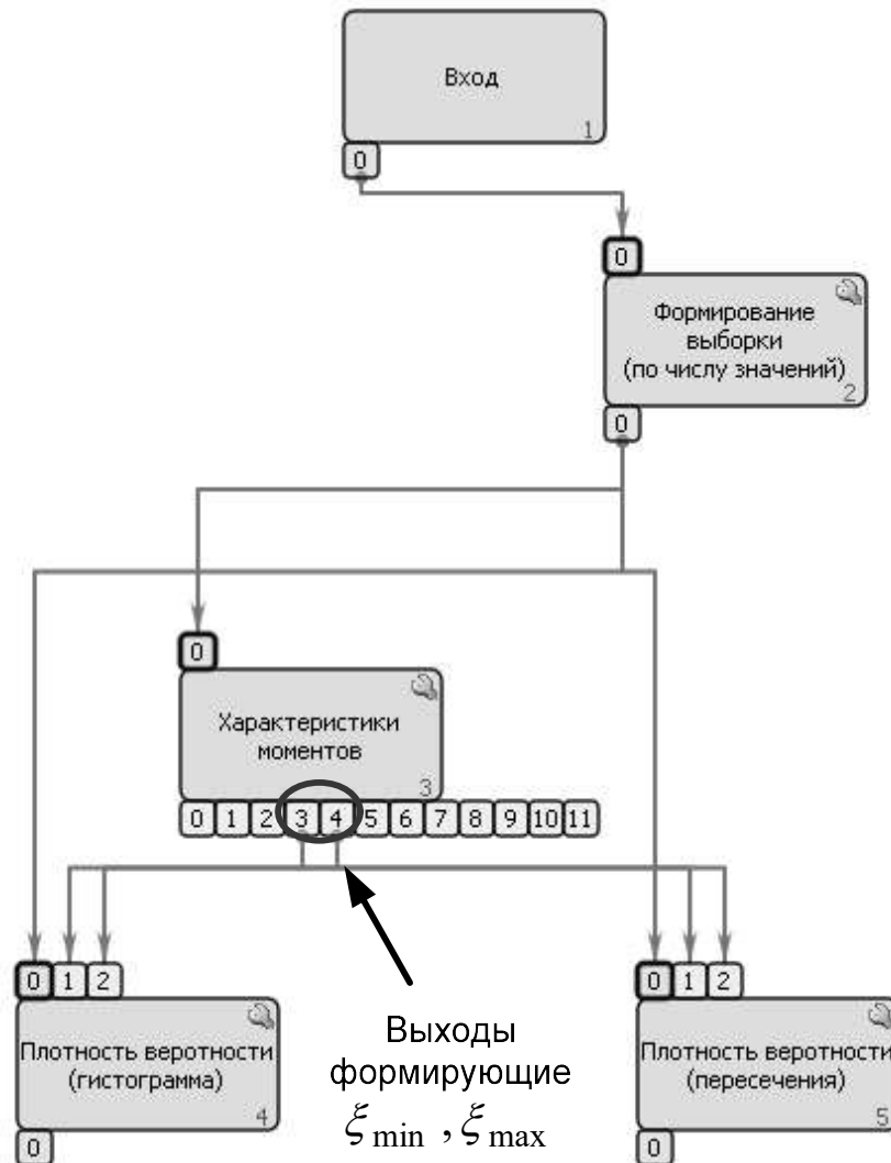
Рисунок 4.13 Реализация процедуры оценивания плотности по методу гистограмм и с использованием характеристик превышения уровня
