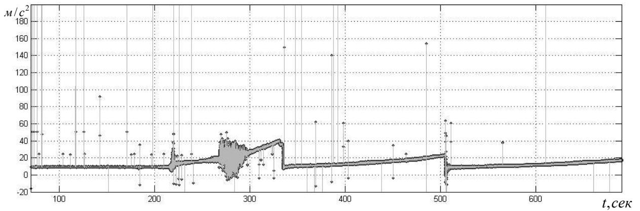
Рисунок 1.10 Графическое представление телеметрической информации, полученной с датчика АЛЕ048 блока «И» ракеты-носителя «Союз-2» с космическим аппаратом «Corot»
