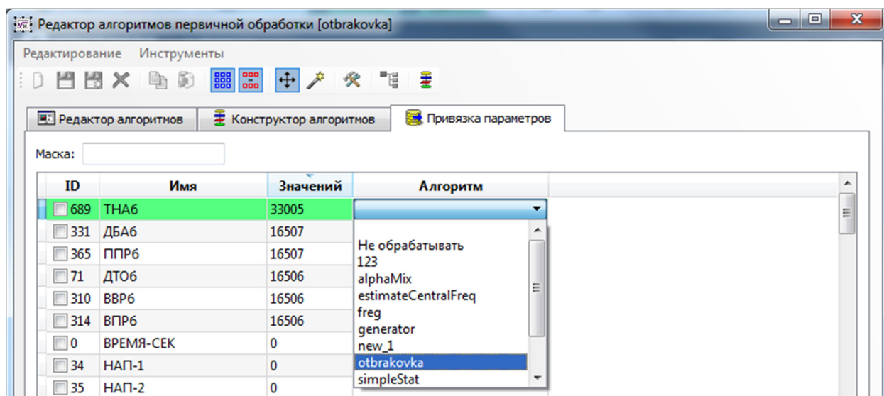
Рисунок 0.1 Привязка параметра ТНАБ к алгоритму «Otbrakovka».
