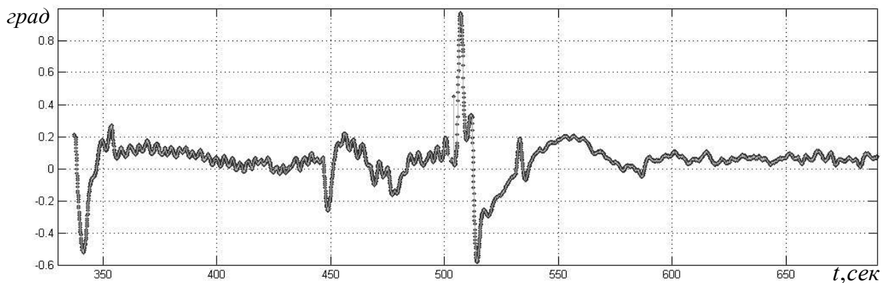
Рисунок 1.13 Графическое представление функционального параметра, поступающего с датчика KEАФ.45-020А блока «И» ракеты-носителя «Союз-2»
