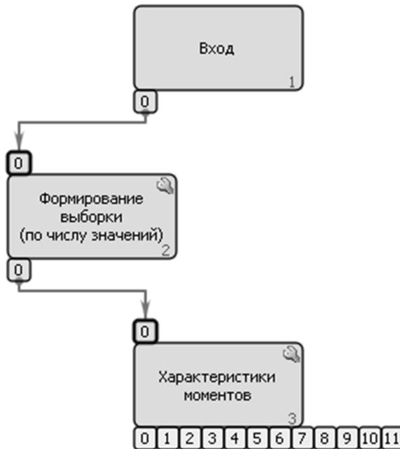
Рисунок 4.10 Реализация процедуры оценивания моментов одномерных распределений телеметрируемого процесса традиционным способом суммирования
