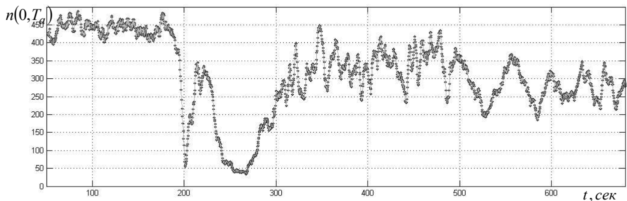
Рисунок 2.2 График изменения числа пересечений нулевого ( N=0 ) уровня траекторией телеметрируемого процесса, получаемого с датчика АЛЕ048 третьей ступени ракеты-носителя «Союз-2»
