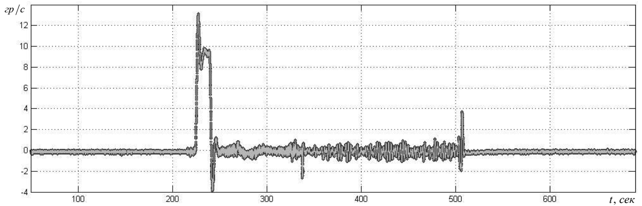
Рисунок 1.14 Графическое представление функционально-диапазонного параметра, поступающего с датчика КЕАФ.34-008А блока «И» ракеты-носителя «Союз-2»
