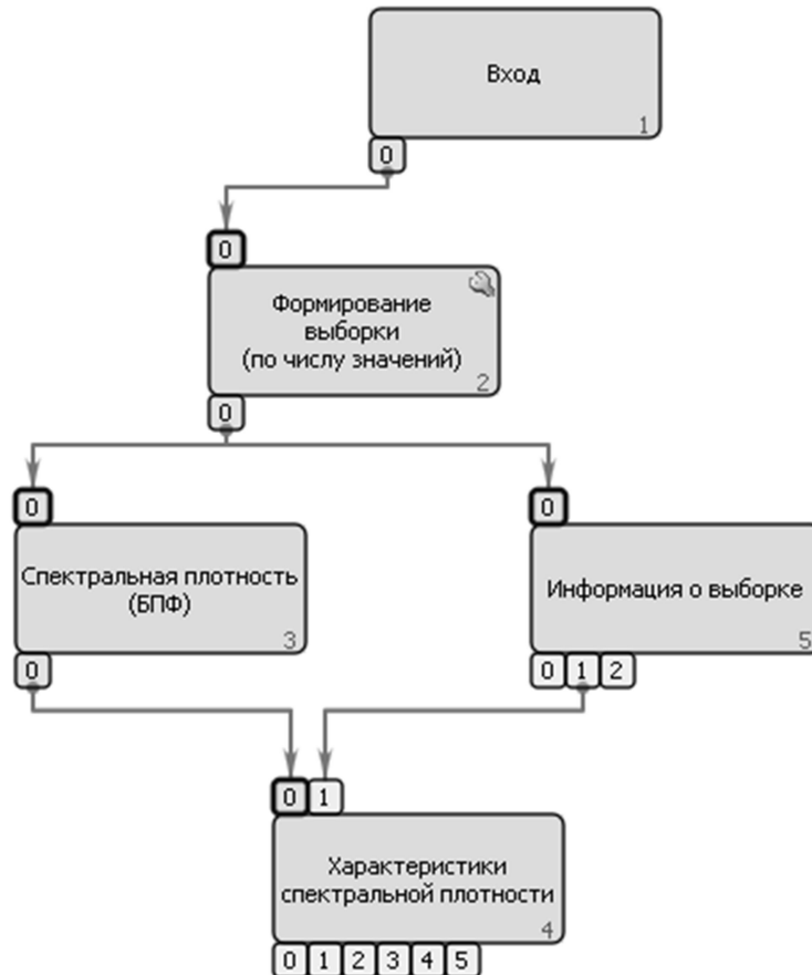
Рисунок 4.7 Реализация процедуры оценивания обобщённых спектрально-корреляционных характеристик телеметрируемых процессов с использованием быстрых преобразований Фурье
