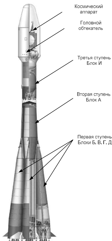
Рисунок 1.2 Упрощенная структурная схема ракеты-носителя «Союз-2» типов 1a, 1б, СТ-А и СТ-Б
