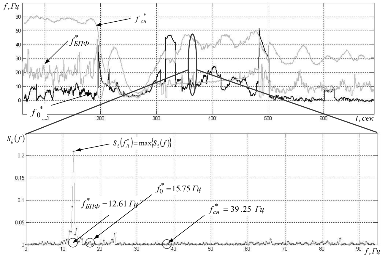
Рисунок 4.9 Результаты работы процедуры оперативного оценивания спектрально-корреляционных характеристик телеметрируемых процессов
