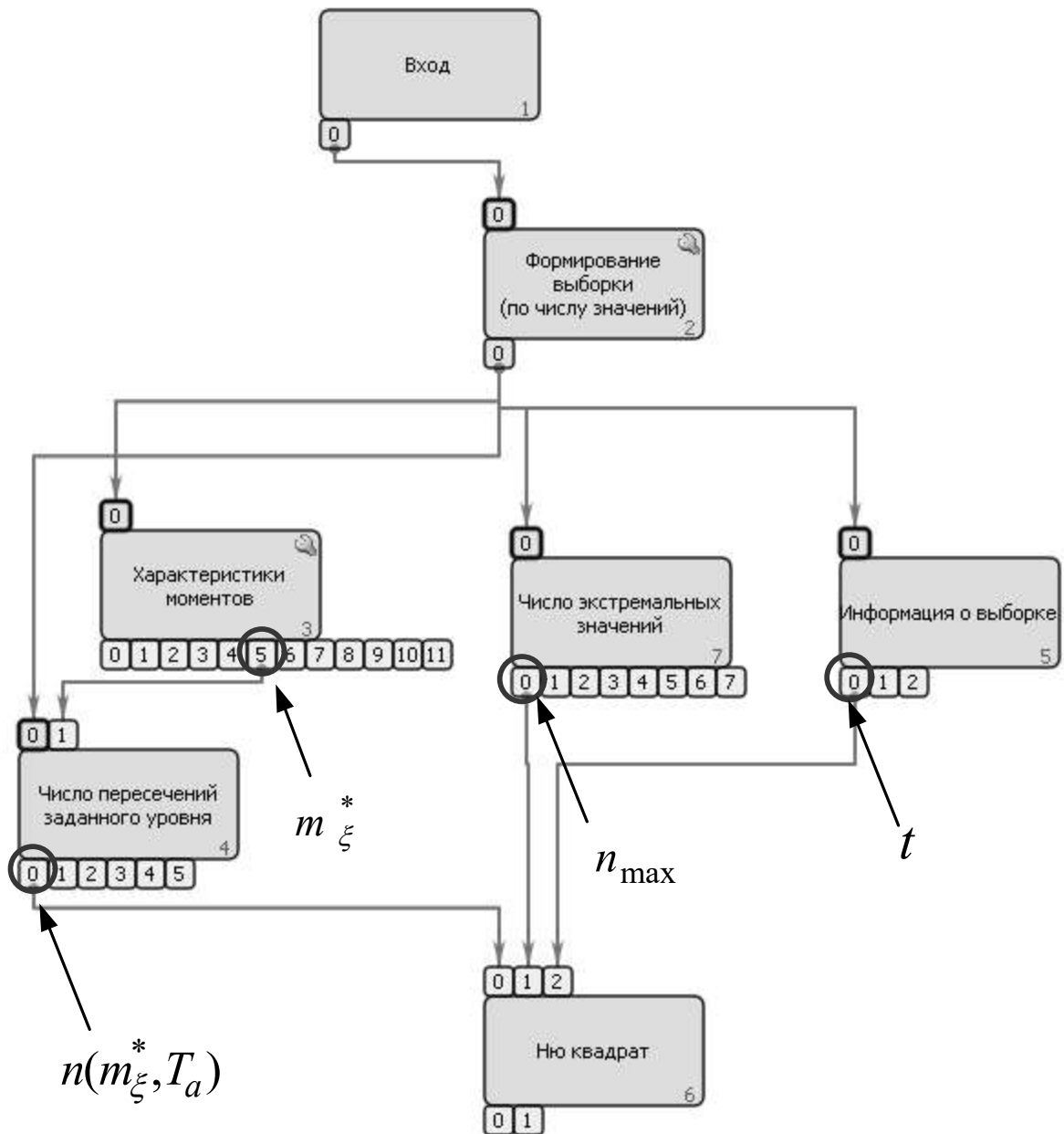
Рисунок 4.11 Реализация процедуры оценивания моментов одномерных распределений телеметрируемого процесса с использованием характеристик превышения уровня
