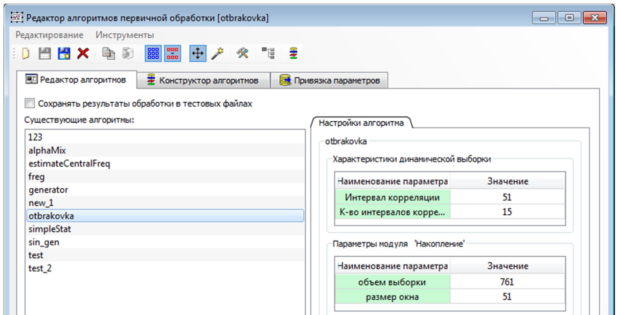
Рисунок 0.8 Отображение настроек выбранного алгоритма.
