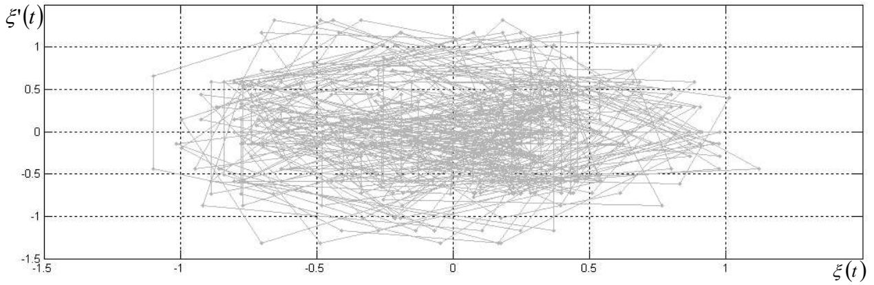
Рисунок 2.14 Характерный вид псевдофазовой траектории телеметрируемого процесса, получаемого с датчика АЛЕ048 третьей ступени ракеты-носителя «Союз-2»
