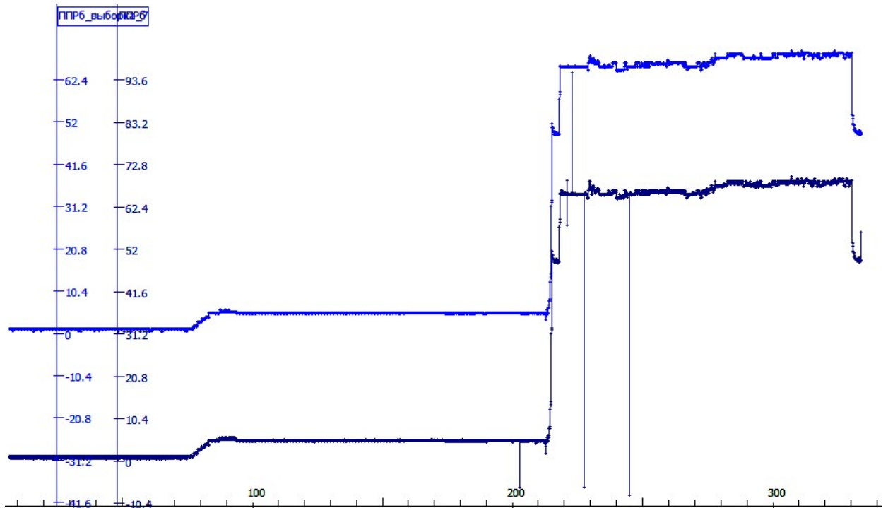
Рисунок 0.4 Результат работы алгоритма отбраковки. Графики параметра ППРб до и после обработки.
