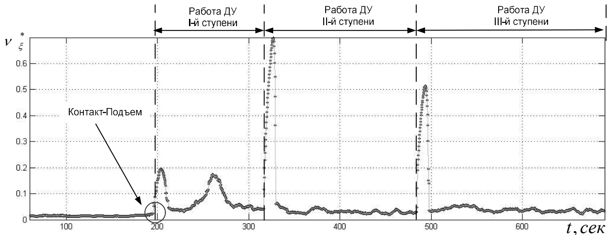
Рисунок 2.9 Изменение оценки коэффициента вариации параметра Осевой Перегрузки, получаемого с датчика АЛЕ048 третьей ступени ракеты-носителя «Союз-2»
