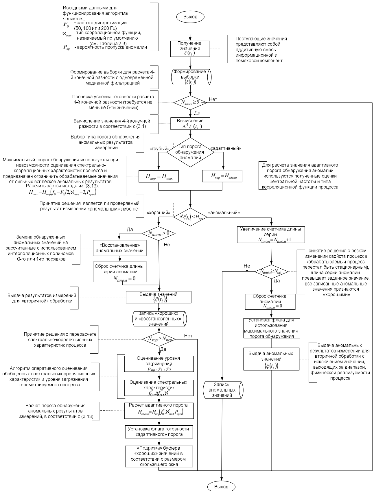
Рисунок 3.1 Блок-схема алгоритма обнаружения и исключения результатов измерений, содержащих аномальную погрешность
