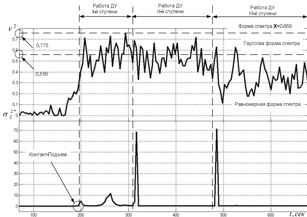
Рисунок 4.17 Сравнение графиков значения метрики (вверху) и дисперсии (внизу) телеметрируемого процесса с датчика осевого ускорения блока «И» ракеты-носителя «Союз-2»
