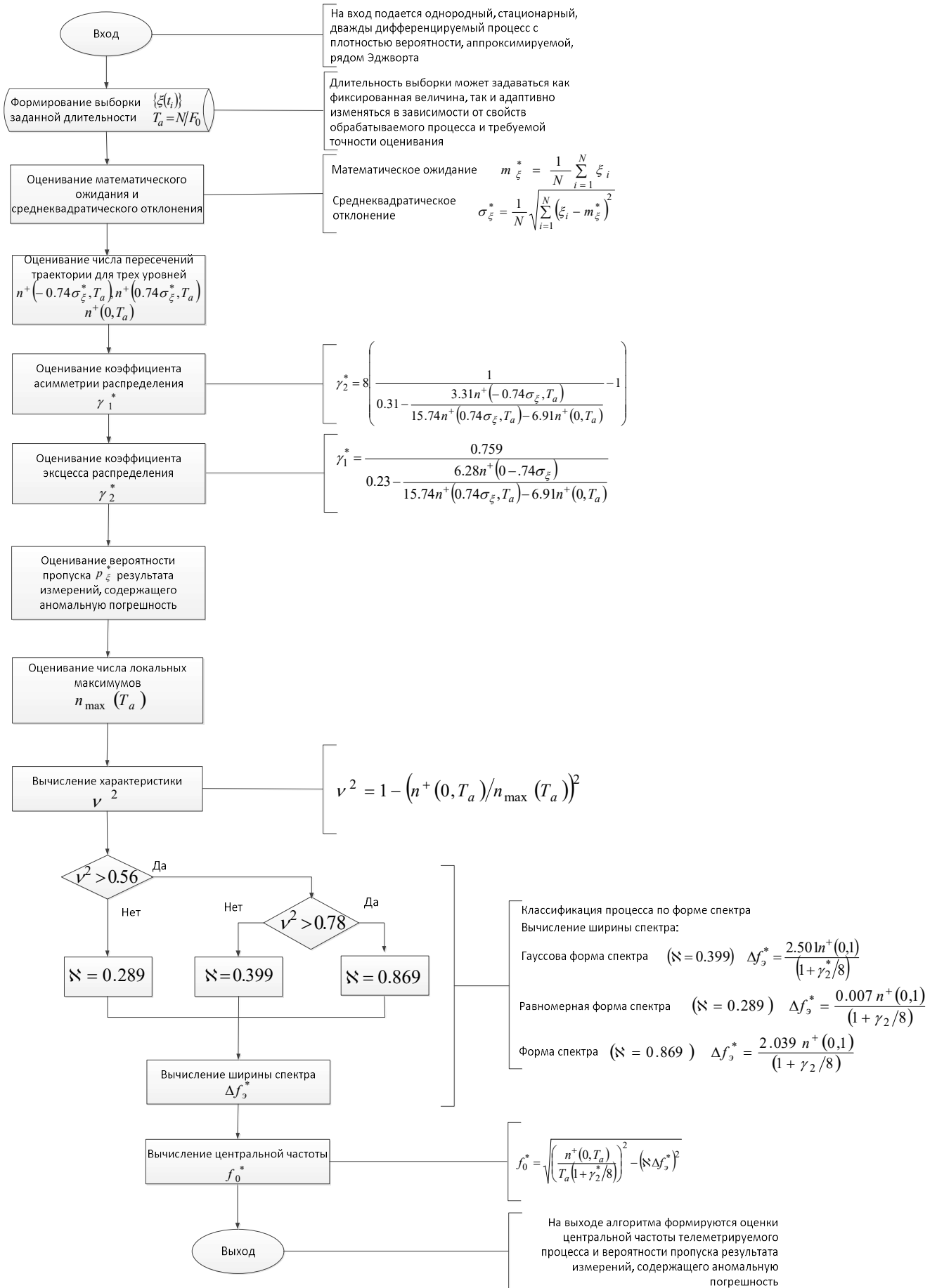
Рисунок 3.7 Блок-схема алгоритма оперативного оценивания величины загрязнения телеметрируемого процесса
