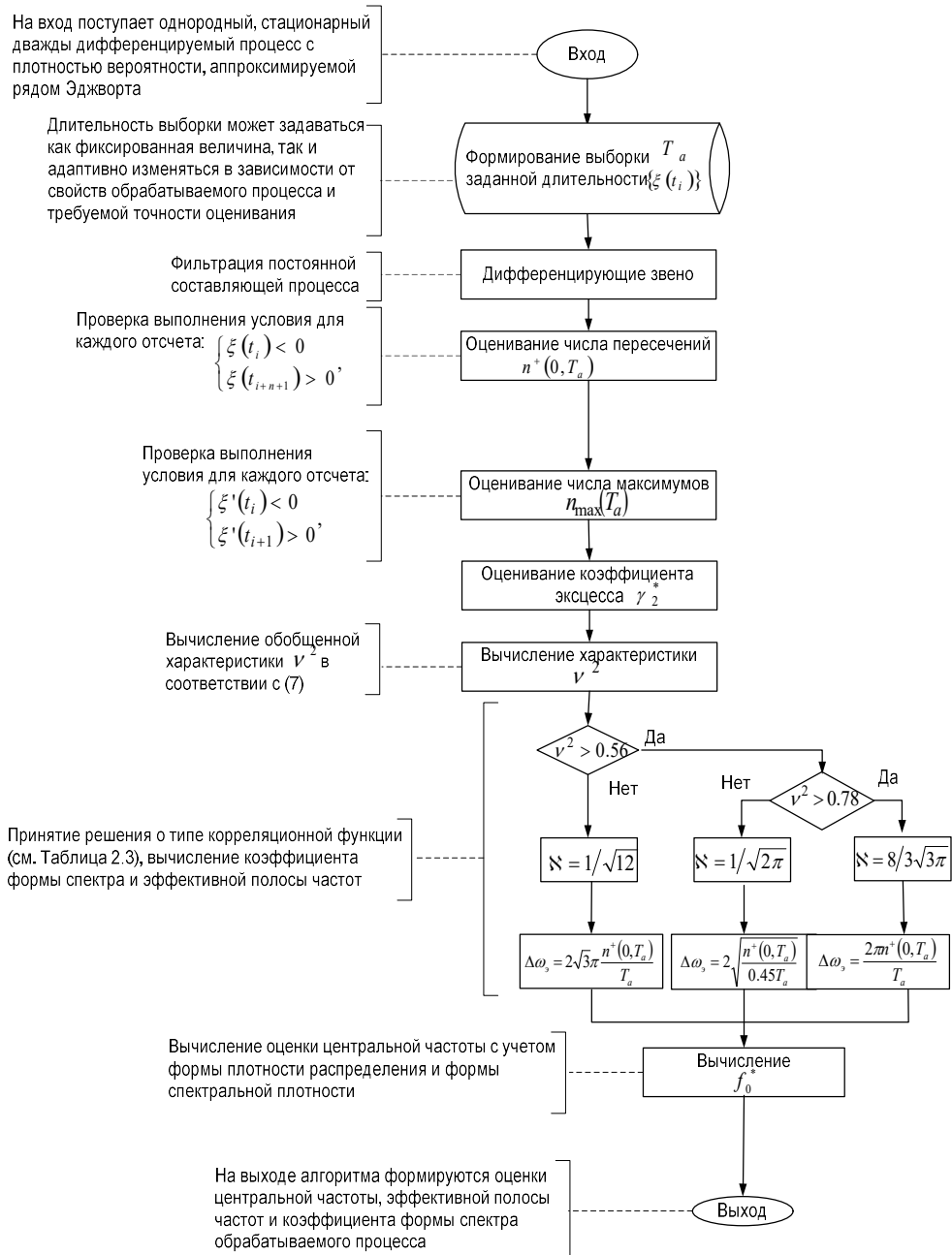
Рисунок 3.4 Блок-схема алгоритма оперативного оценивания обобщенных спектрально-корреляционных характеристик
