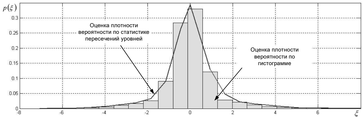
Рисунок 2.16 Сравнение оценок плотности вероятности по методу гистограмм и статистике превышения уровня
