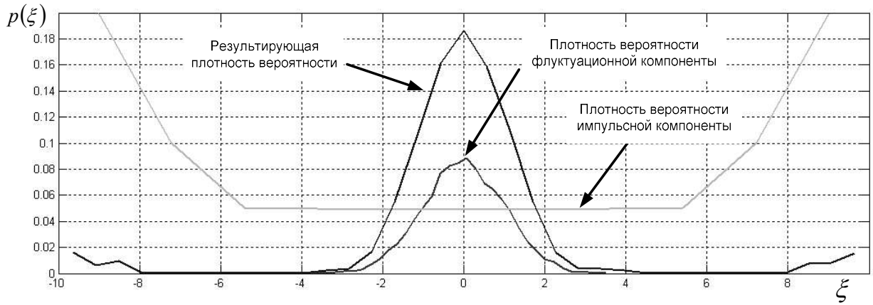
Рисунок 2.21 Результаты численного моделирования плотности вероятности, состоящей из смеси гауссовой и арксинусной компонент
