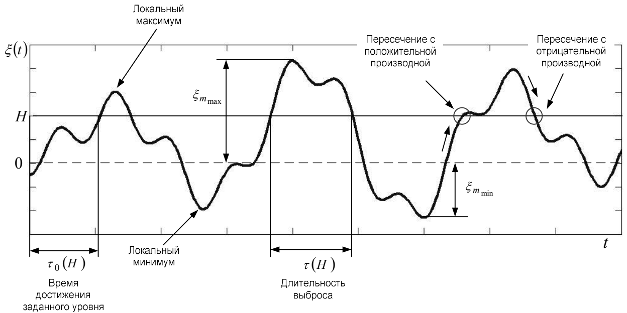
Рисунок 2.1 Характеристики типа «превышения уровня» траектории случайных процессов
