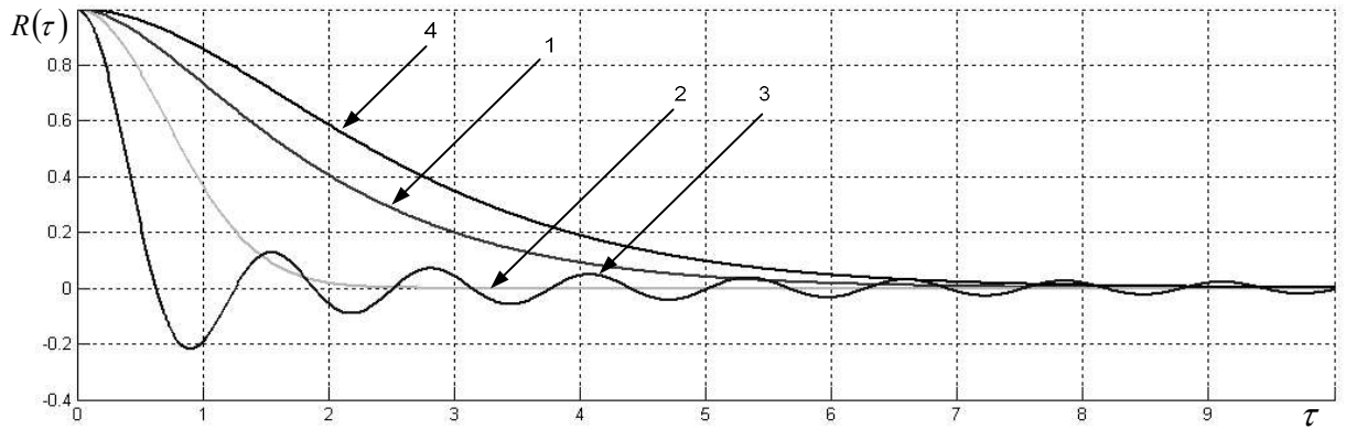
Рисунок 2.36 Графическое представление основных типов однопараметрических нормированных корреляционных функций
