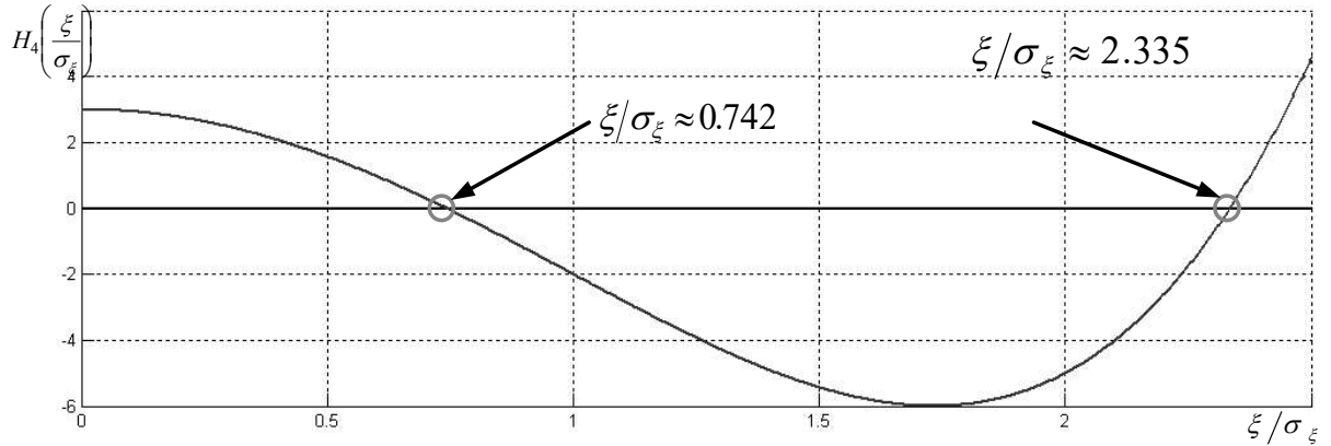
Рисунок 2.28 Корни полинома Эрмита четвертой степени
