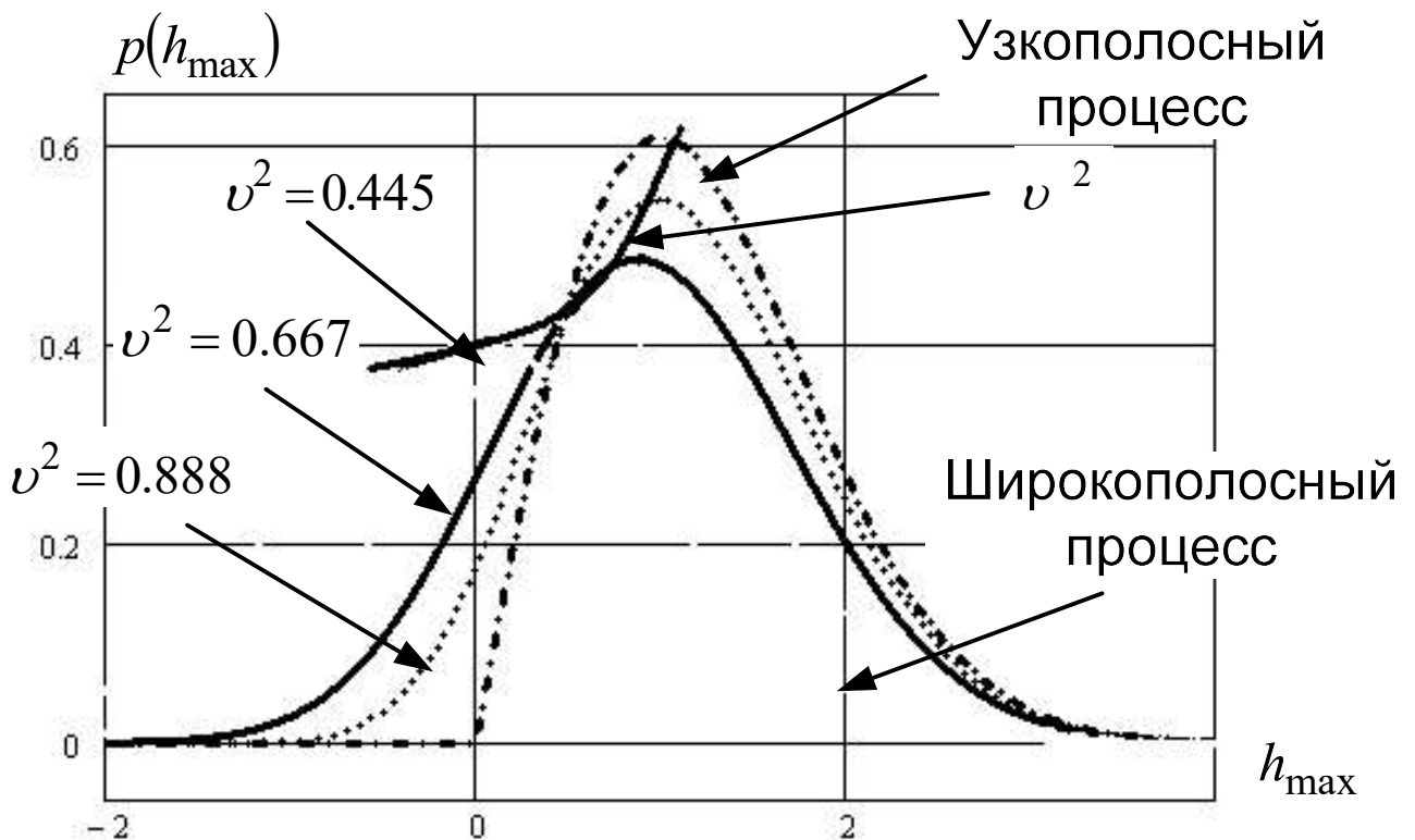
Рисунок 2.35 Плотность вероятности высоты локальных максимумов при различных значениях характеристики \nu^2
