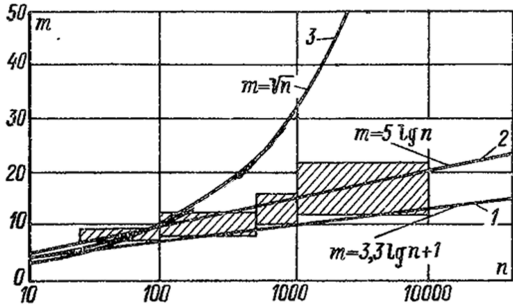
Рисунок 2.12 Оптимальное число столбцов гистограммы по различным критериям выборки различного объема
