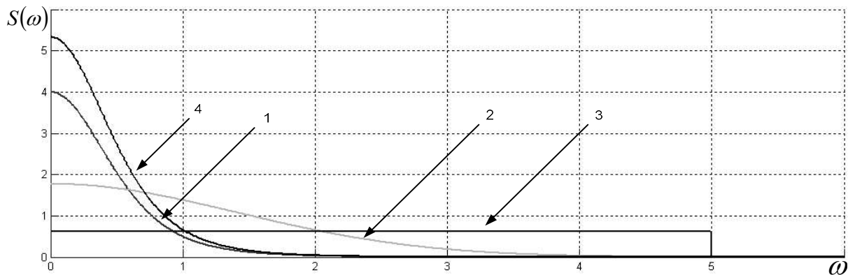
Рисунок 2.37 Графическое представление основных типов однопараметрических нормированных спектральных плотностей
