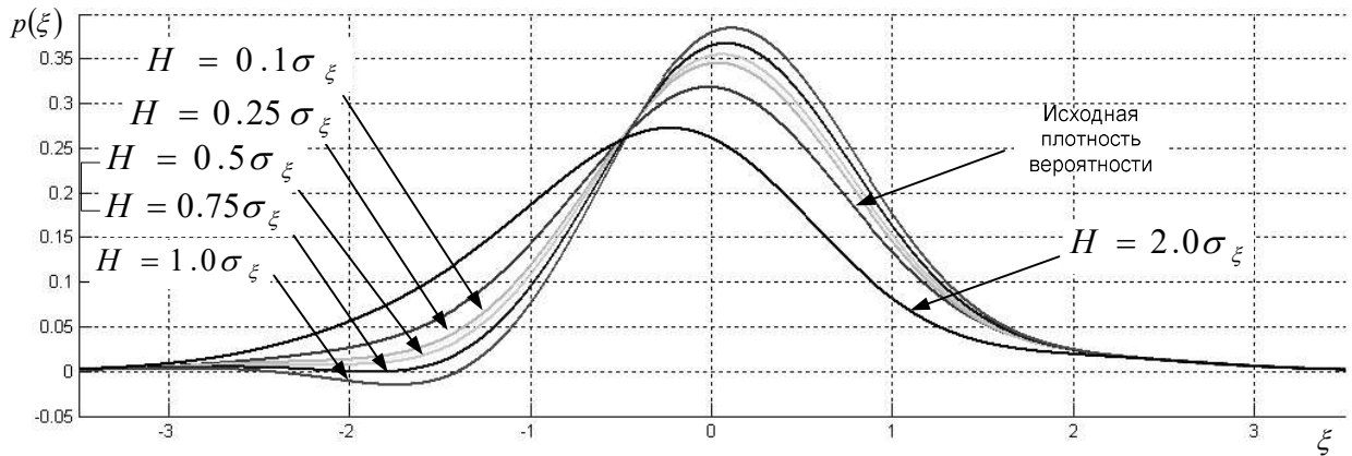
Рисунок 2.26 Изменение аппроксимации плотности вероятности рядом Эджворта при значениях H < 2.5\sigma_\xi
