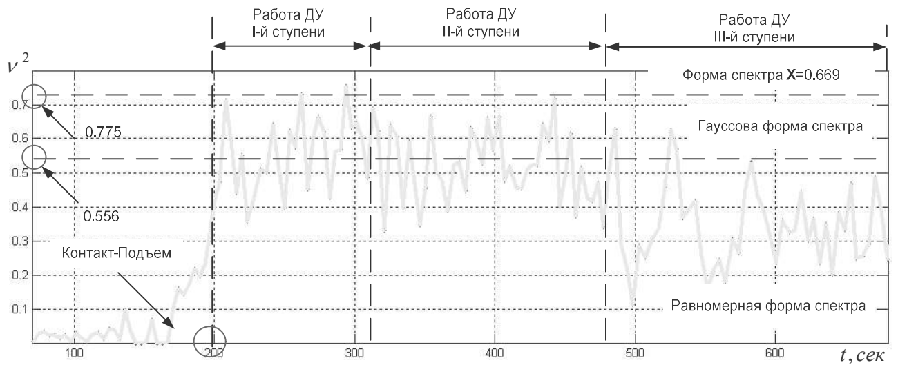
Рисунок 2.38 График изменения оценки характеристики \nu^2 параметра Осевой Перегрузки, получаемого с датчика АЛЕ048 третьей ступени ракеты-носителя «Союз-2»
