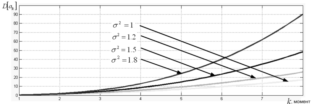
Рисунок 2.6 Графики изменения дисперсии оценки начального момента в зависимости от его порядка
