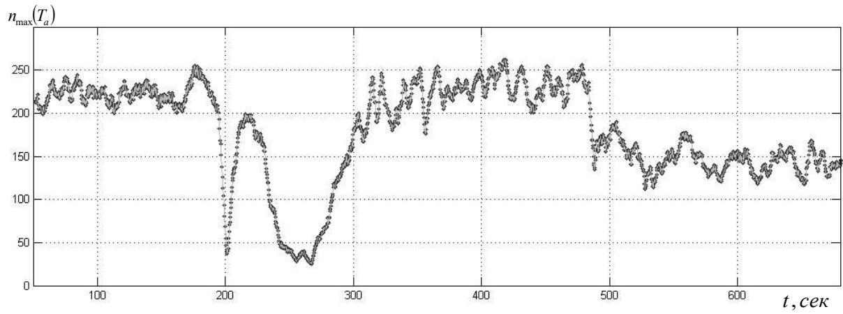
Рисунок 2.3 График изменения числа локальных максимумов траектории телеметрируемого процесса, получаемого с датчика АЛЕ048 третьей ступени ракеты-носителя «Союз-2»
