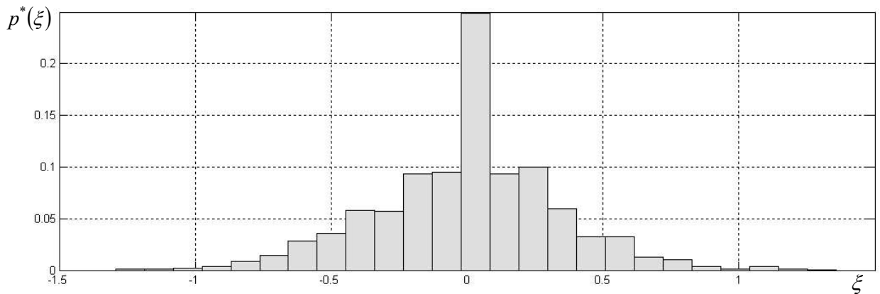
Рисунок 2.13 Характерный вид плотности вероятности параметра ОП, получаемого с датчика АЛЕ048 третьей ступени ракеты-носителя «Союз-2» во время работы двигательной установки 2-й ступени (385-390 с)
