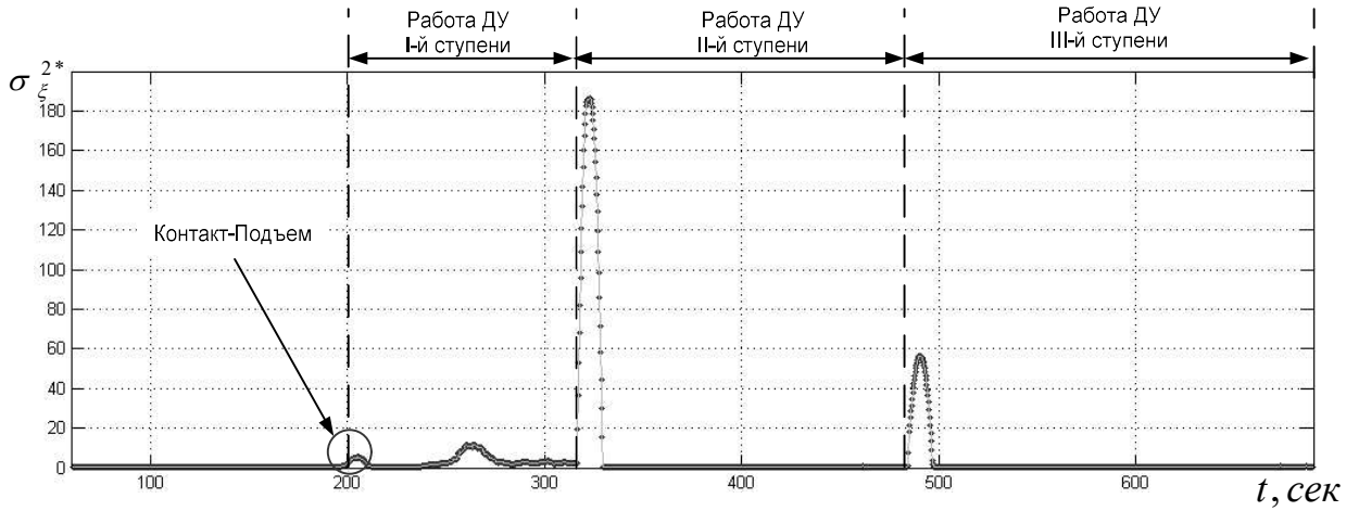
Рисунок 2.8 Изменение оценки дисперсии параметра Осевой Перегрузки, получаемого с датчика АЛЕ048 третьей ступени ракеты-носителя «Союз-2»
