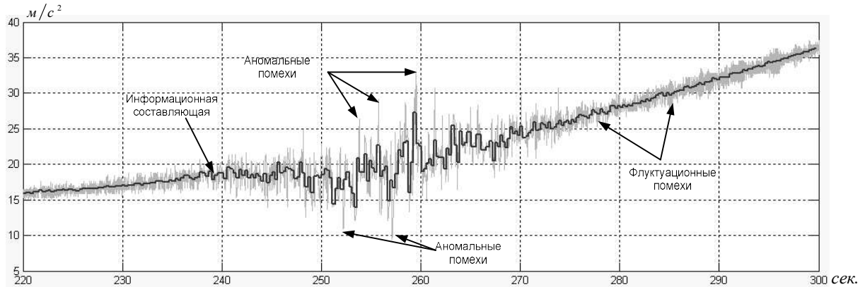
Рисунок 1.8 Графическое представление различных видов помех, воздействующих на телеметрическую информацию ракет-носителей «Союз-2».
