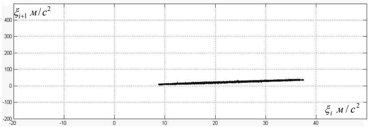
Рисунок 4.16 Псевдофазовый портрет телеметрируемого процесса с датчика осевого ускорения блока «И» ракеты-носителя «Союз-2» после применения алгоритма обнаружения результатов измерений, содержащих аномальную погрешность
