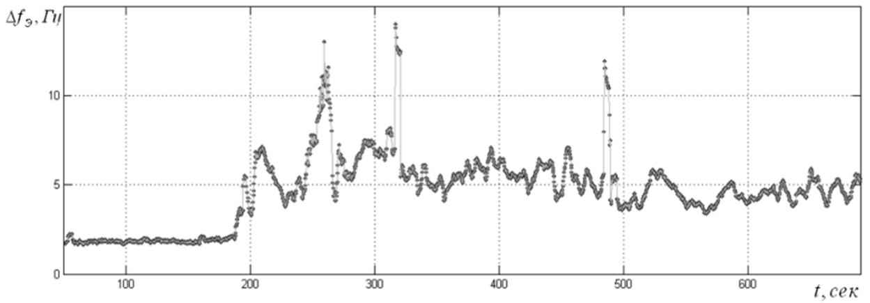
Рисунок 2.33 График изменения оценки эффективной полосы частот для параметра Осевой Перегрузки, получаемого с датчика АЛЕ048 третьей ступени ракеты-носителя «Союз-2»
