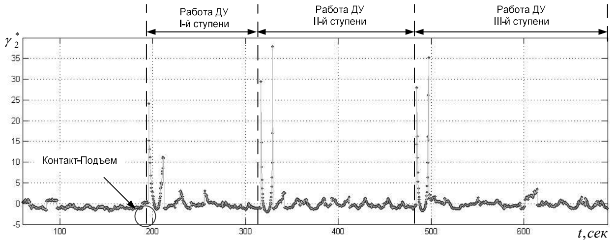
Рисунок 2.11 Изменение оценки коэффициента эксцесс параметра ОП, получаемого с датчика АЛЕ048 третьей ступени ракеты-носителя «Союз-2»
