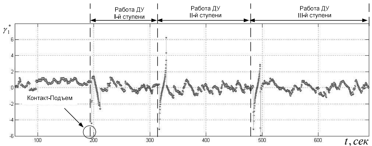
Рисунок 2.10 Изменение оценки коэффициента асимметрии параметра ОП, получаемого с датчика АЛЕ048 третьей ступени ракеты-носителя «Союз-2»
