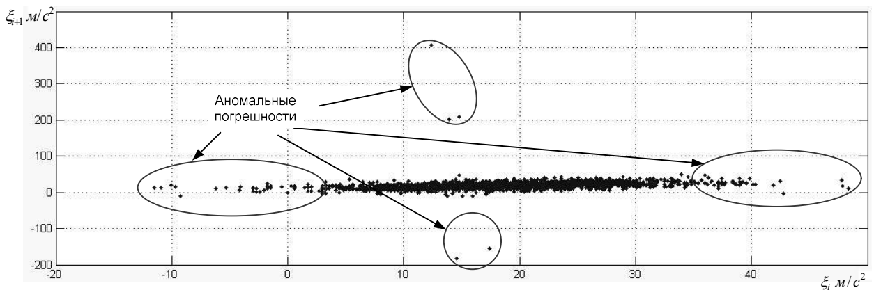
Рисунок 1.12 Диаграмма рассеивания телеметрической информации, полученной с датчика АЛЕ048 блока «И» ракеты-носителя «Союз-2» с космическим аппаратом «Сорот»
