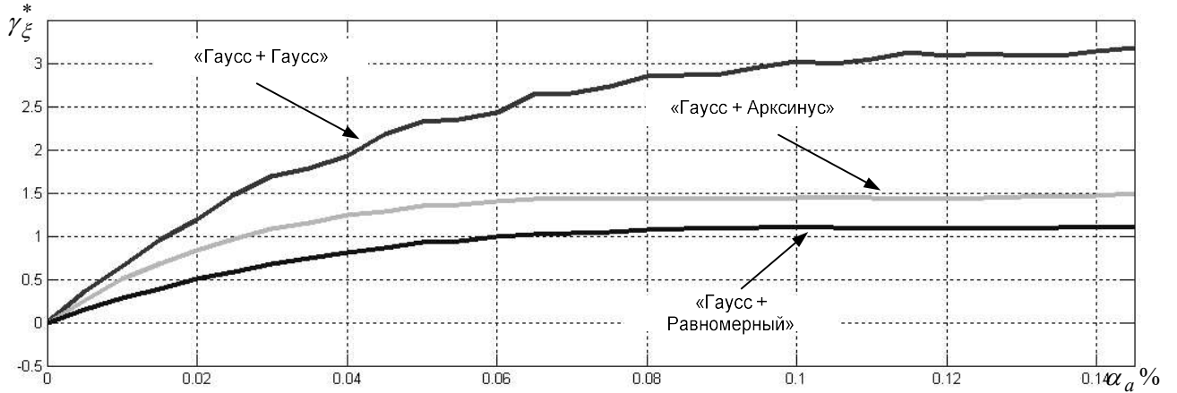
Рисунок 2.24 Графики изменения значения коэффициента эксцесса в зависимости уровня загрязнения телеметрируемого процесса
