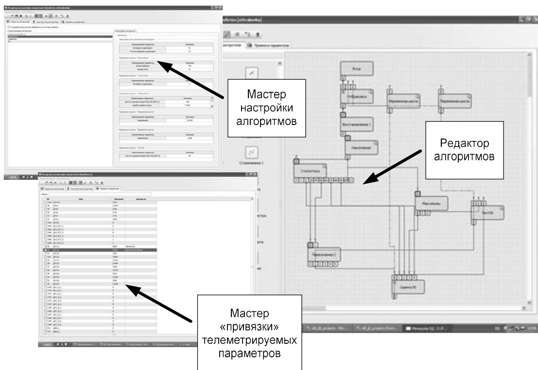
Рисунок 4.1 Общий вид «Конструктор алгоритмов» оперативной подготовки телеметрической информации
