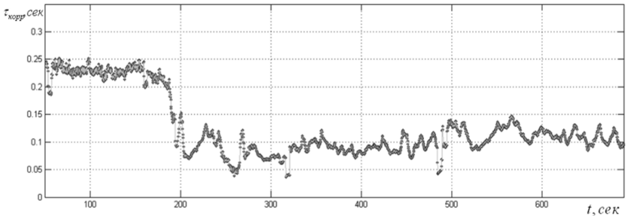
Рисунок 2.34 График изменения оценки интервала корреляции для параметра Осевой Перегрузки, получаемого с датчика АЛЕ048 третьей ступени ракеты-носителя «Союз-2»
