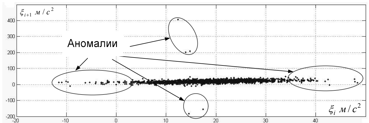
Рисунок 4.15 Псевдофазовый портрет телеметрируемого процесса с датчика осевого ускорения блока «И» ракеты-носителя «Союз-2» до применения алгоритма обнаружения результатов измерений, содержащих аномальную погрешность
