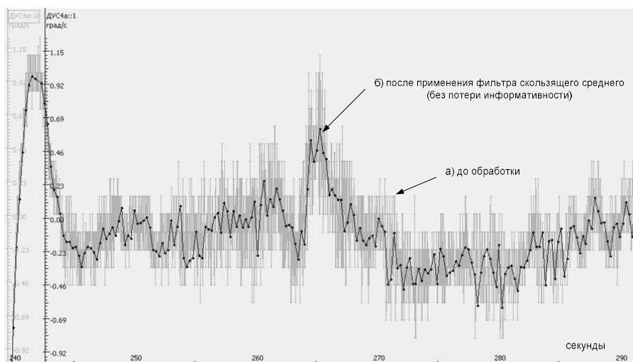
Рисунок 1.17 Телеметрическая информация, поступающая с датчика угловой скорости блока А: а) до обработки объем измерений составлял 104566 байт, б) после применения алгоритмов сглаживания - 2151 бит
