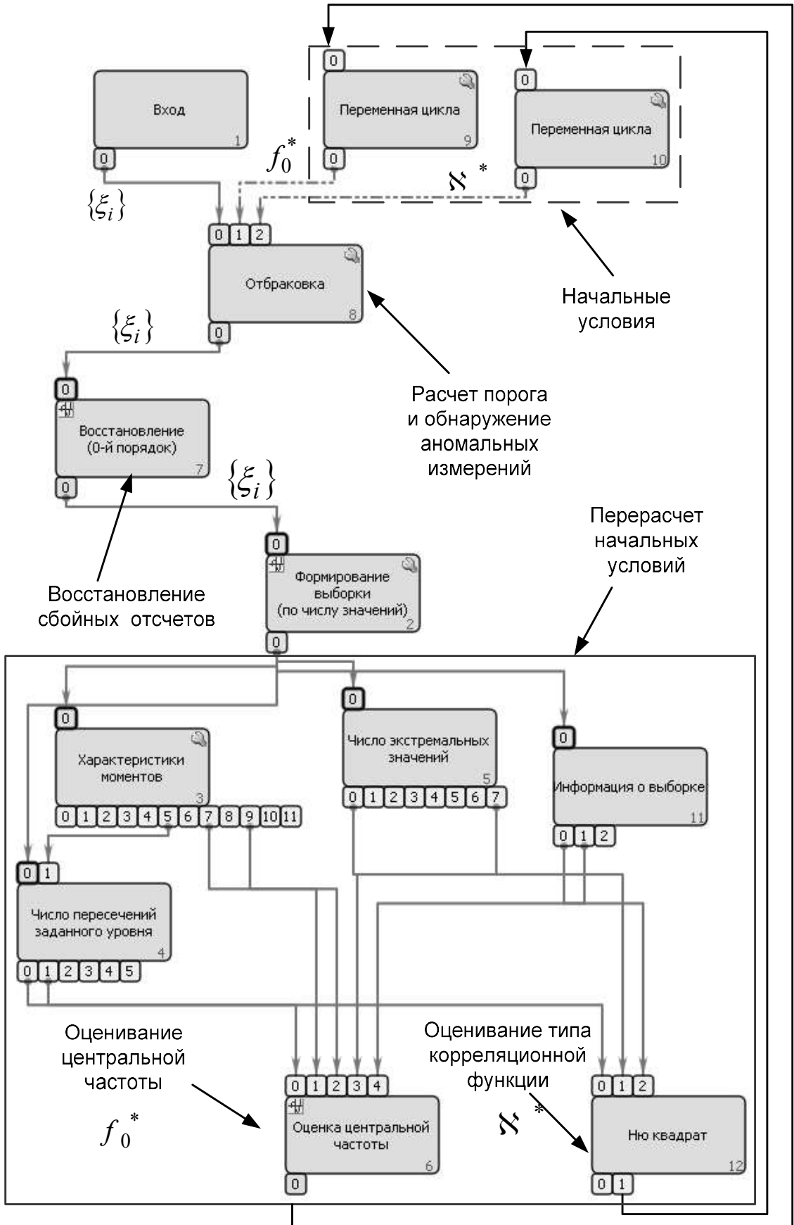
Рисунок 4.14 Реализация алгоритма обнаружения и исключения результатов измерений, содержащих аномальную погрешность
