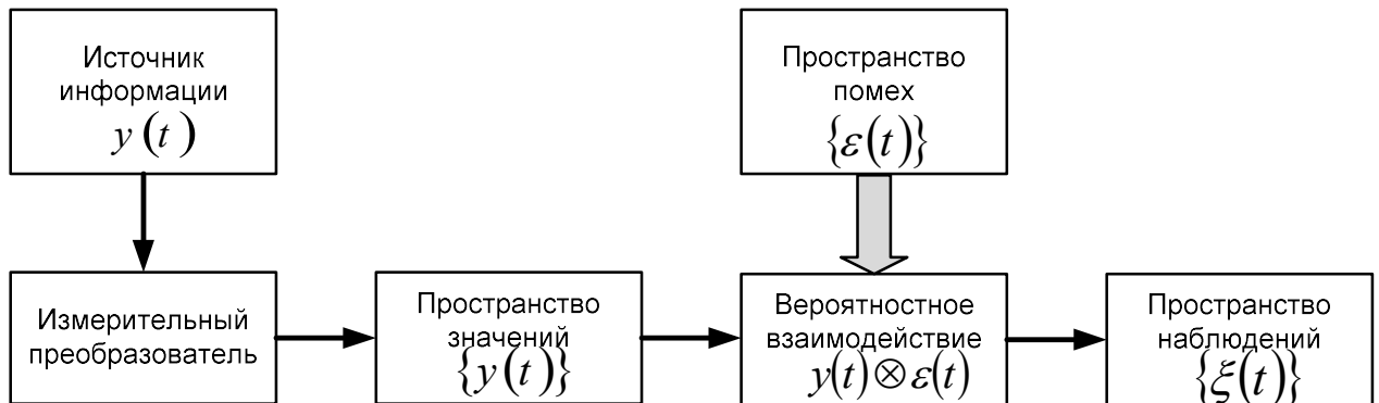
Рисунок 1.7 Обобщенная формализованная модель получения и передачи телеметрической информации
