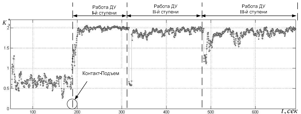
Рисунок 2.17 График изменения оценки коэффициента энтропии, параметра Осевая Перегрузка, получаемого с датчика АЛЕ048 третьей степени ракеты-носителя «Союз-2»
