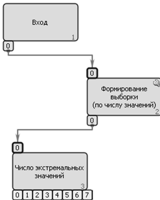
Рисунок 4.6 Реализация процедуры подсчета числа экстремальных значений телеметрируемого процесса
