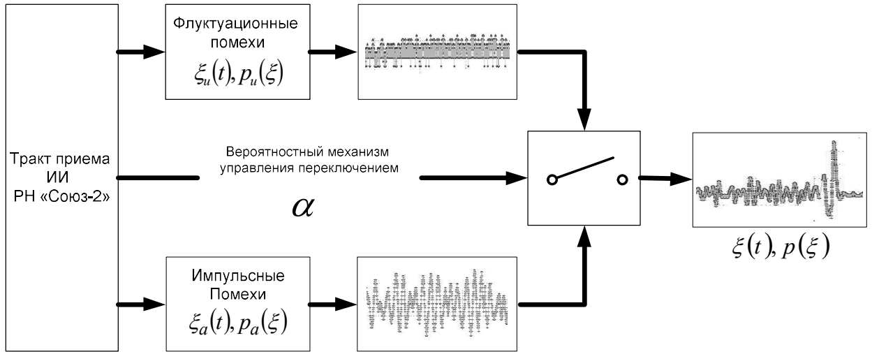
Рисунок 2.19 Упрощенная схема формирования телеметрируемых процессов
