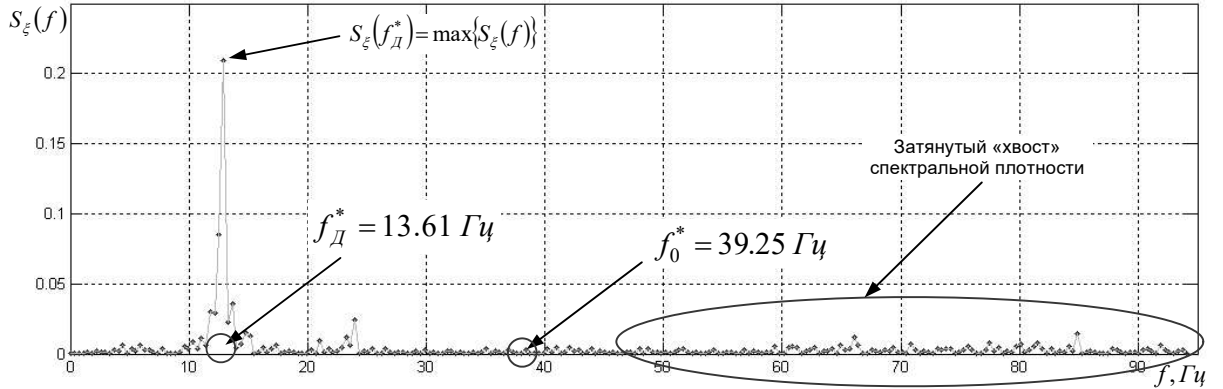
Рисунок 3.3 Оценка спектральной плотности параметра Осевой Перегрузки, получаемого с датчика АЛЕ048 третьей ступени РН «Союз-2», и смещение оценки f_0^*
