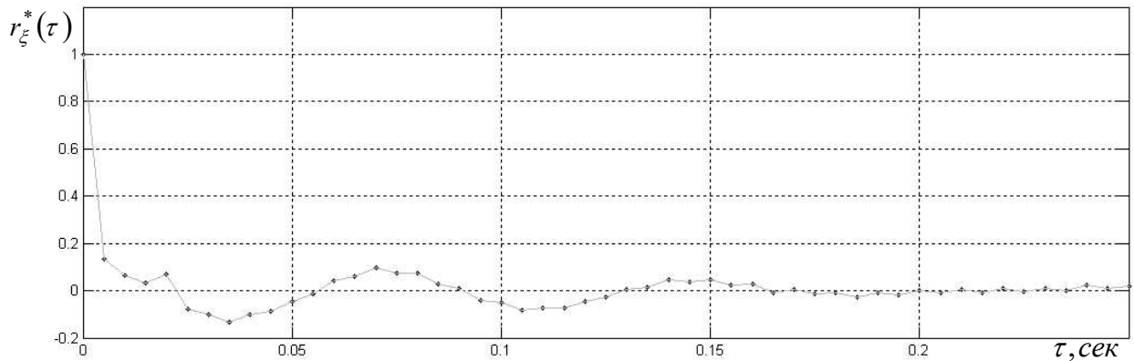
Рисунок 2.30 Характерный вид оценки нормированной корреляционной функции телеметрируемого параметра ракеты-носителя «Союз-2»
