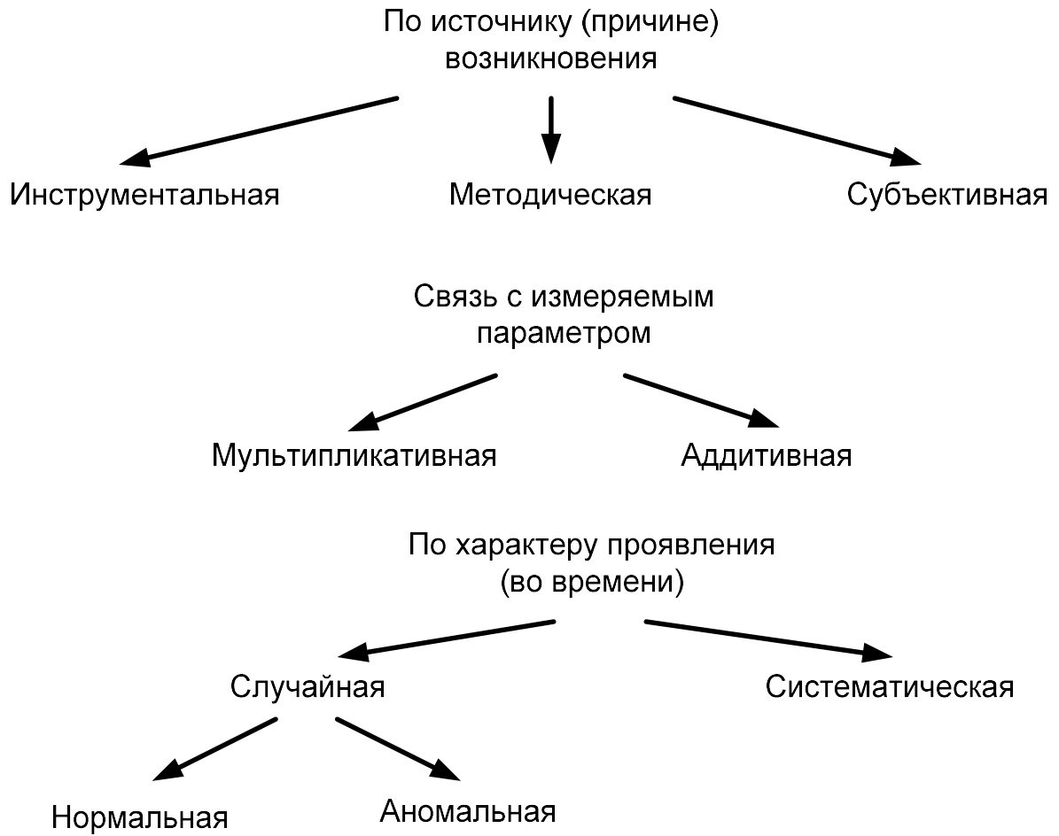
Рисунок 1.9 Классификация погрешностей телеметрической информации
