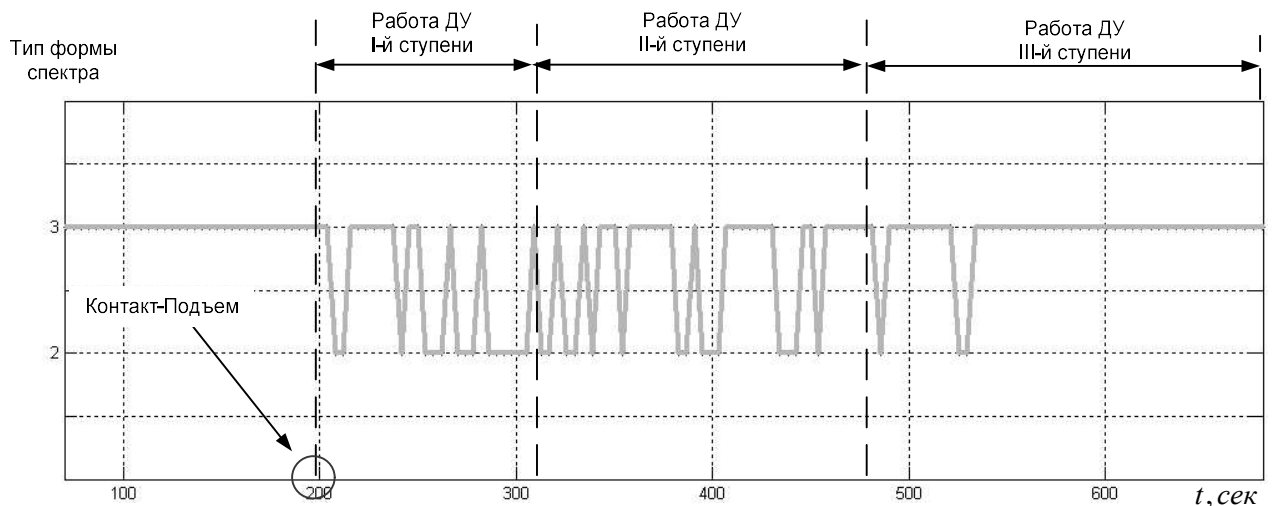
Рисунок 2.39 График изменения типа корреляционной функции и спектральной плотности параметра Осевой Перегрузки, получаемого с датчика АЛЕ048 третьей ступени ракеты-носителя «Союз-2»
