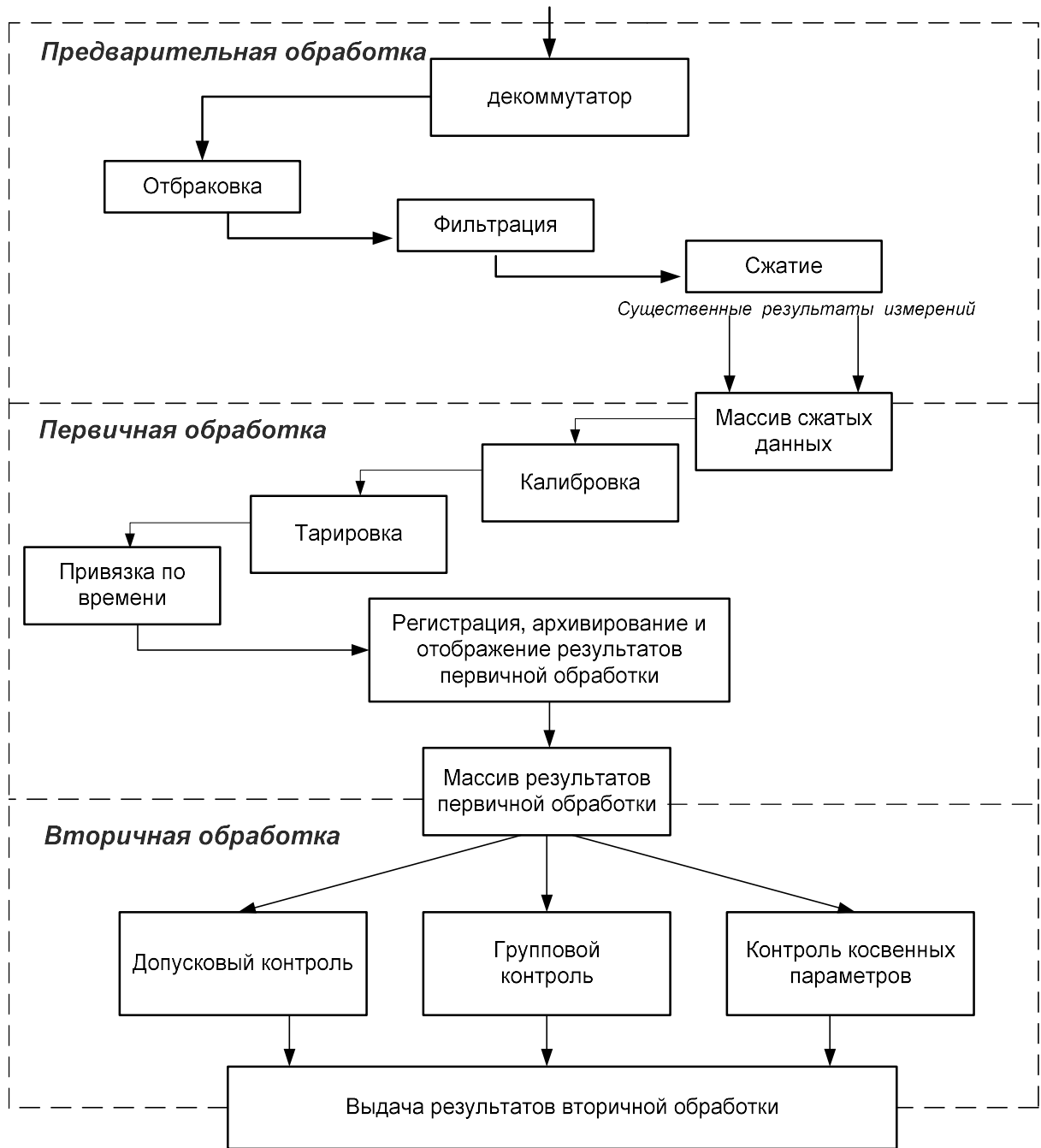
Рисунок 1.16 Схема существующего алгоритма обработки поступающей телеметрической информации семейства ракет-носителей «Союз-2»
