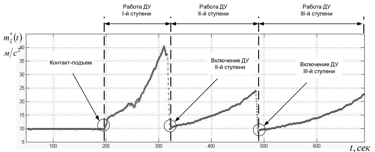
Рисунок 2.7 Изменение оценки математического ожидания параметра ОП, получаемого с датчика АЛЕ048 третьей ступени ракеты-носителя «Союз-2»
