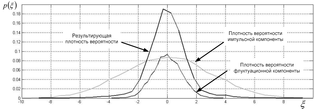
Рисунок 2.20 Результаты численного моделирования плотности вероятности, состоящей из двух гауссовых компонент
