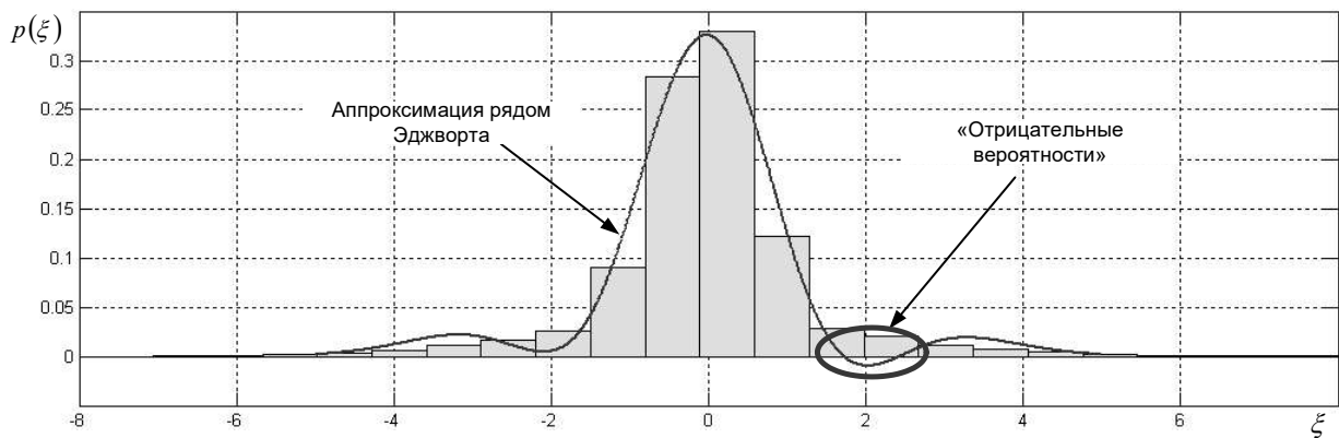
Рисунок 2.25 Аппроксимация плотности вероятности рядом Эджворта
