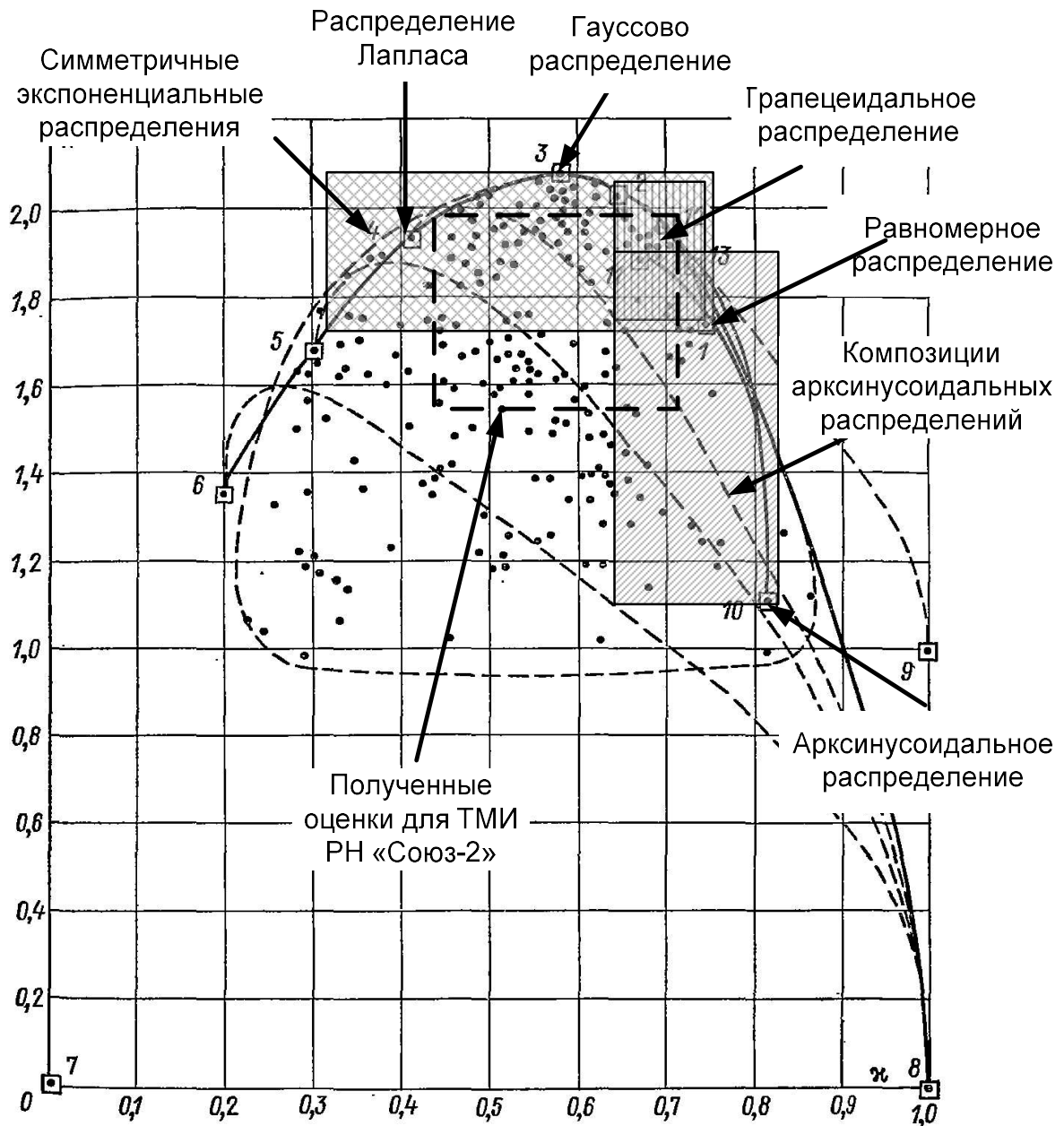
Рисунок 2.18 Результаты оценивания значения энтропии и коэффициента формы полученных оценок p^*(\xi)
