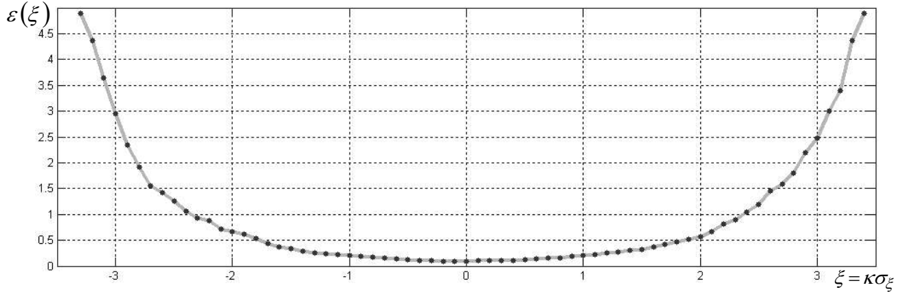
Рисунок 2.15 График изменения значения величины относительной погрешности оценивания плотности вероятности с использованием характеристик превышения уровня
