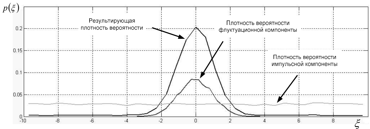
Рисунок 2.22 Результаты численного моделирования плотности вероятности, состоящей из смеси гауссовой и равномерной компонент
