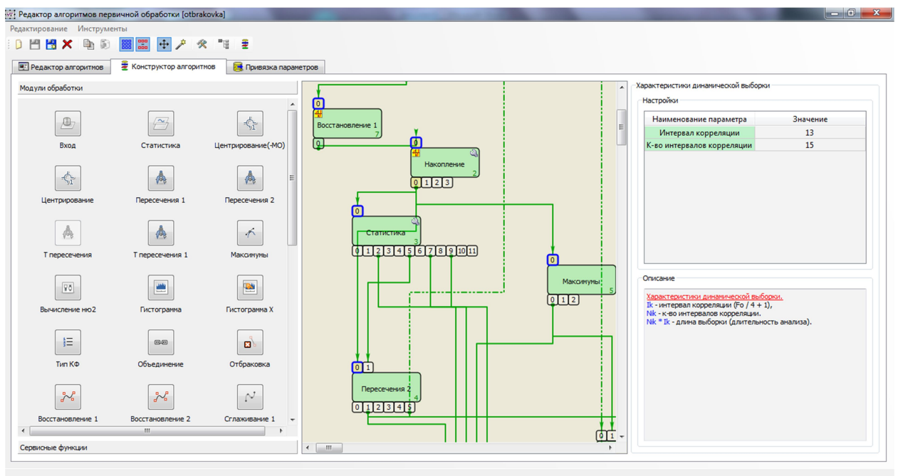
Рисунок 0.9 Вкладка «Конструктор алгоритмов» «Редактора алгоритмов первичной обработки данных».
