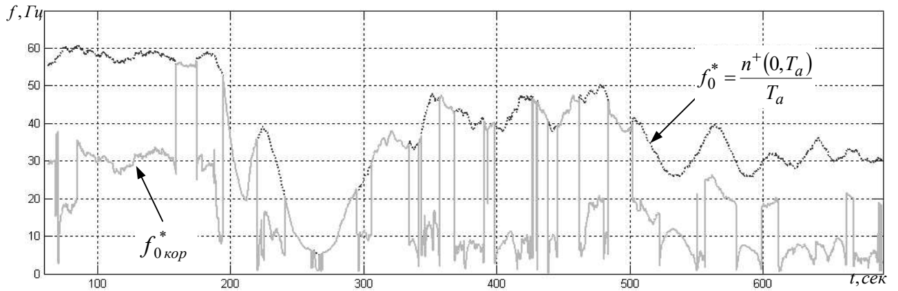
Рисунок 3.5 Графики оценки центральной частоты полученной методом типа «счетчик нулей» и ее скорректированная оценка
