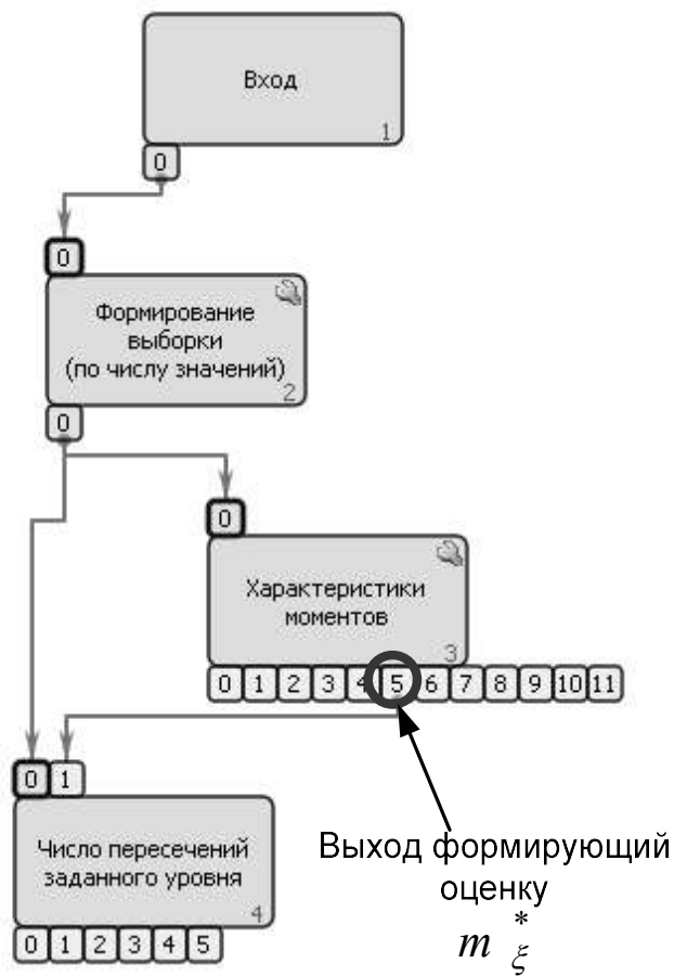
Рисунок 4.4 Реализация алгоритма оценивания средней частоты телеметрируемого процесса «счетчиком нулей»
