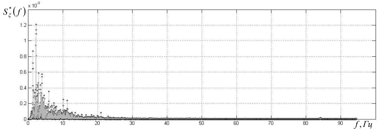
Рисунок 2.31 Характерный вид оценки нормированной спектральной плотности телеметрируемого параметра ракеты-носителя «Союз-2»
