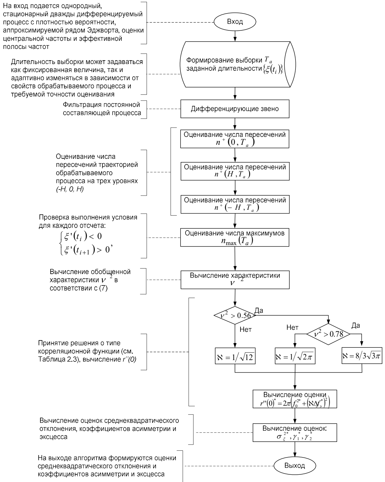
Рисунок 3.6 Блок-схема алгоритма оперативного оценивания характеристик моментов одномерных распределений
