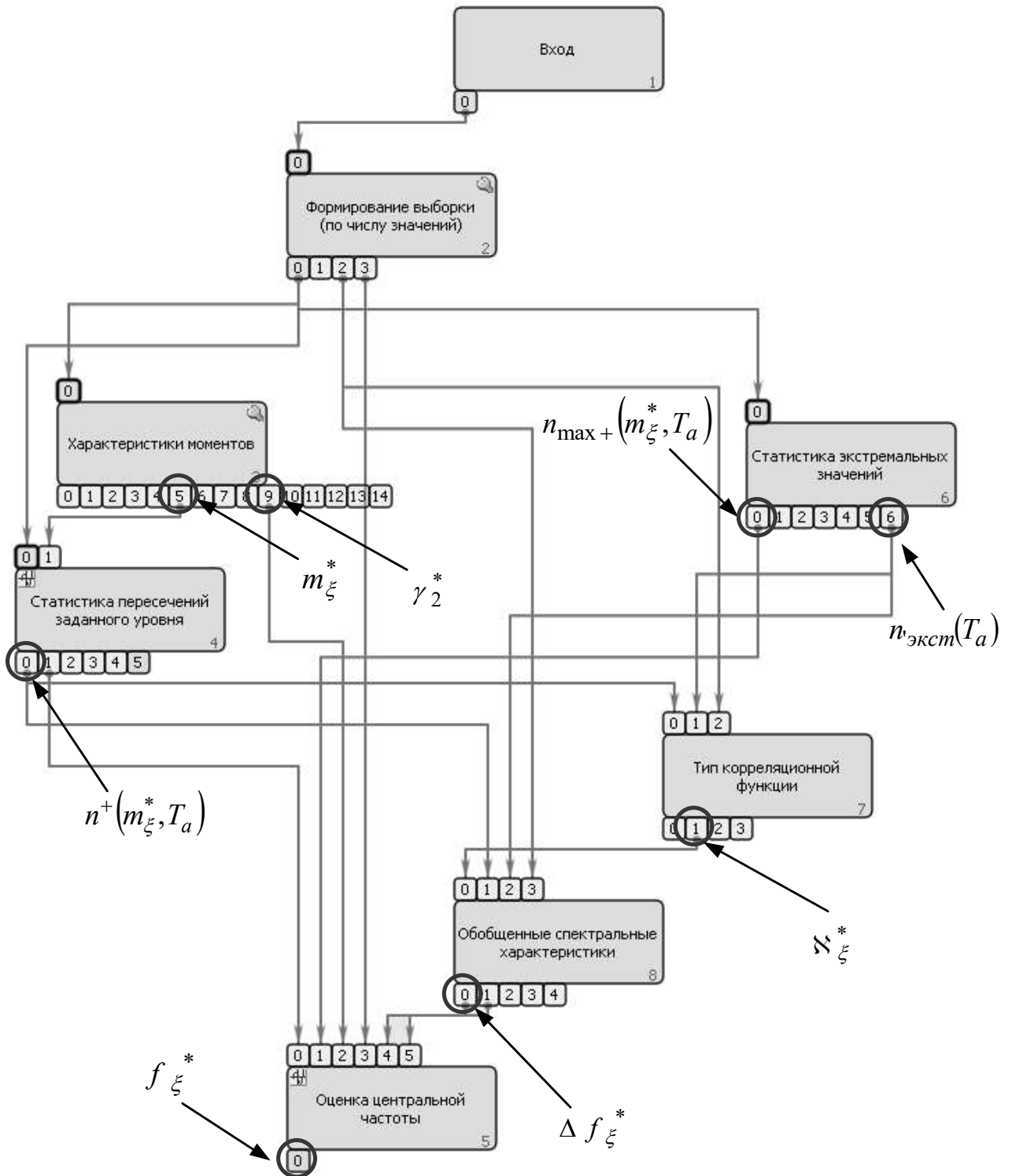
Рисунок 4.8 Реализация процедуры оперативного оценивания обобщённых спектрально-корреляционных характеристик телеметрируемых процессов с использованием характеристик превышения уровня
