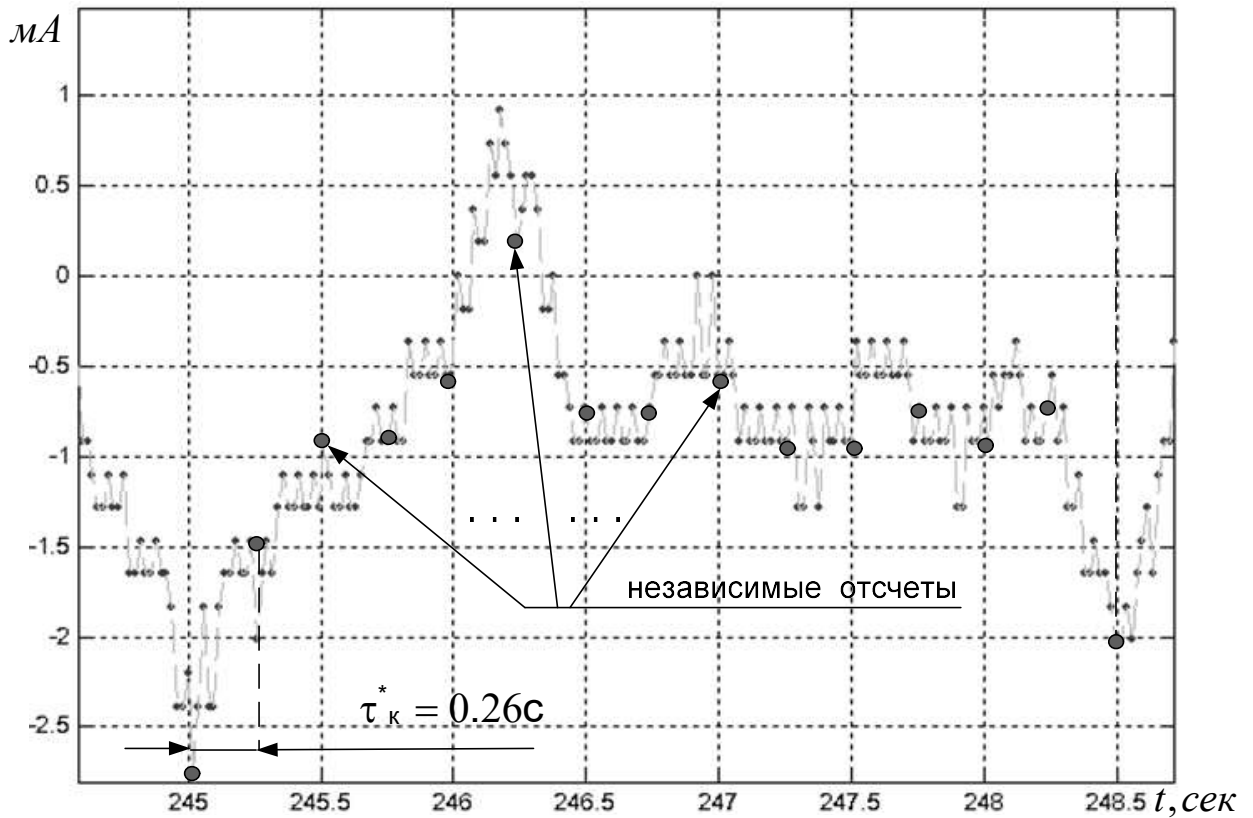
Рисунок 4.3 Графическая интерпретация формирования выборки по независимым отсчетам, полученной с датчика тока управления рулевыми машинами первой ступени; частота опроса 100 Гц.
