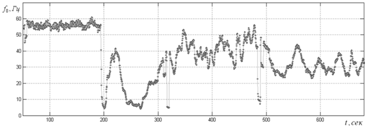
Рисунок 2.32 График изменения оценки центральной частоты для параметра Осевая Перегрузка, получаемого с датчика АЛЕ048 третьей ступени ракеты-носителя «Союз-2»
