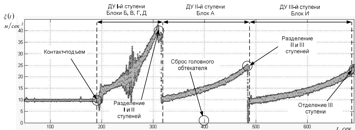
Рисунок 1.3 Графическое представление телеметрируемого параметра Осевой Перегрузки системы управления, полученного в ходе запуска ракеты-носителя «Союз-2» с космическим аппаратом «Corot» 27 декабря 2006 года
