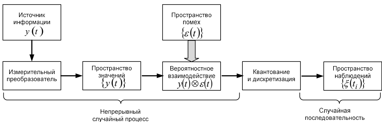
Рисунок 1.18 Обобщенная модель формирования и передачи телеметрической информации семейства ракет-носителей «Союз 2»
