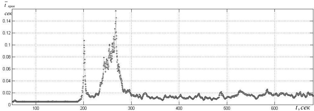
Рисунок 2.5 График изменения среднего времени превышения нулевого уровня ( H=0 ) траекторией телеметрируемого процесса, получаемого с датчика АЛЕ048 третьей ступени ракеты-носителя «Союз-2»
