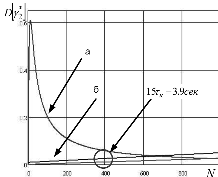
Рисунок 4.12 График изменения дисперсии оценки эксцесса в зависимости от объема выборки для параметра с частотой опроса 100 Гц а) традиционные методы б) с использованием характеристик превышения уровня (для процессов с различной формой спектра)
