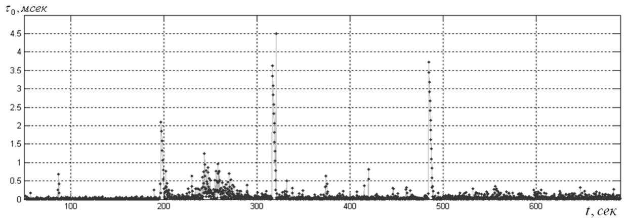
Рисунок 2.4 График изменения времени первого достижения заданного уровня ( H=0 ) траекторией телеметрируемого процесса, получаемого с датчика АЛЕ048 третьей ступени ракеты-носителя «Союз-2»
