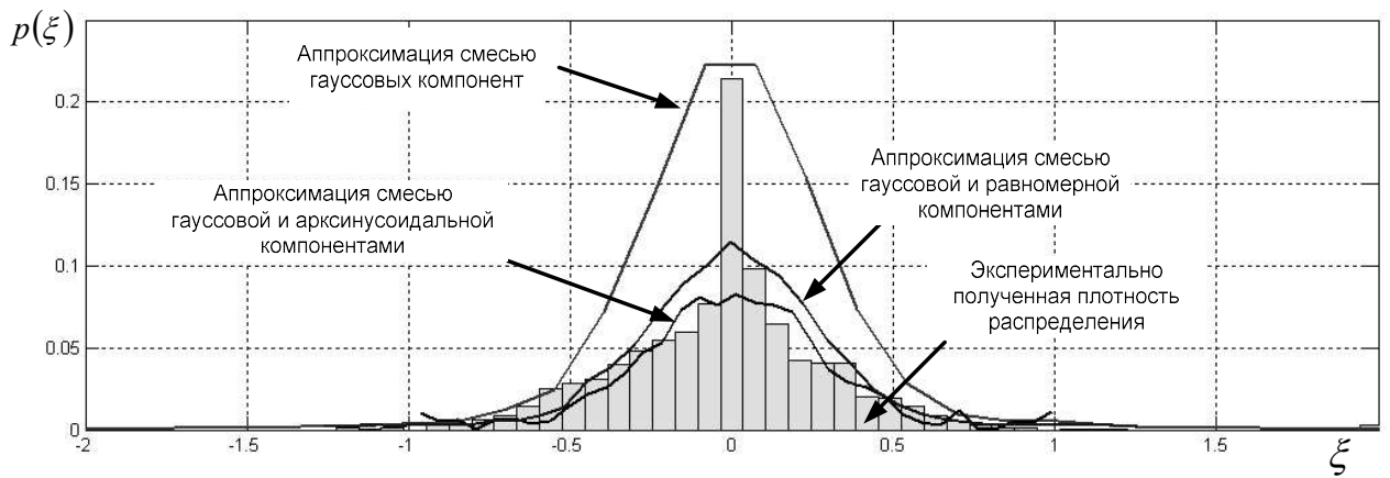
Рисунок 2.23 Аппроксимация плотности вероятности телеметрической информации, полученной с датчика АЛЕ048 третьей ступени ракеты-носителя «Союз-2»
