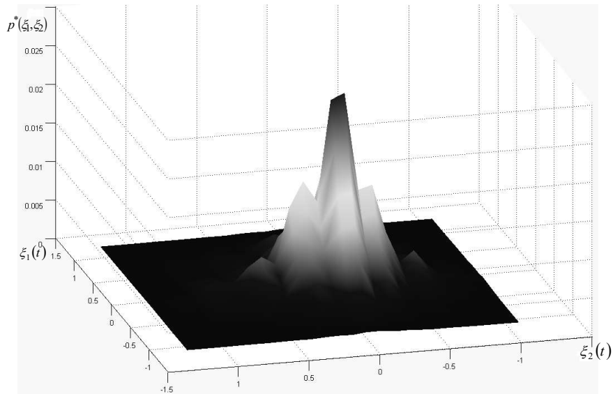
Рисунок 2.29 Оценка двумерной плотности вероятности параметра Осевой Перегрузки, получаемого с датчика АЛЕ048 третьей ступени ракеты-носителя «Союз-2» во время работы двигательной установки 3-й ступени (560-580 с)
