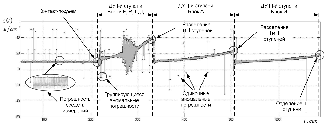
Рисунок 1.11 Виды погрешностей телеметрической информации, встречающихся при обработке телеметрической информации ракет-носителей «Союз-2»
