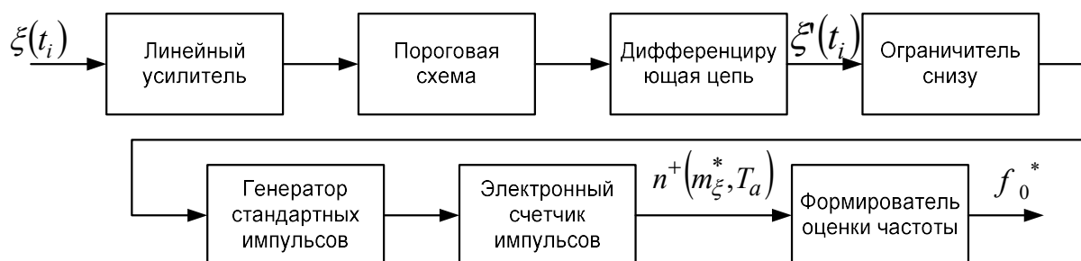
Рисунок 3.2 Измеритель частоты сигнала методом «счетчика нулей»
