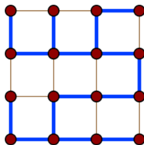
Рисунок 1. Пример остовного дерева.
